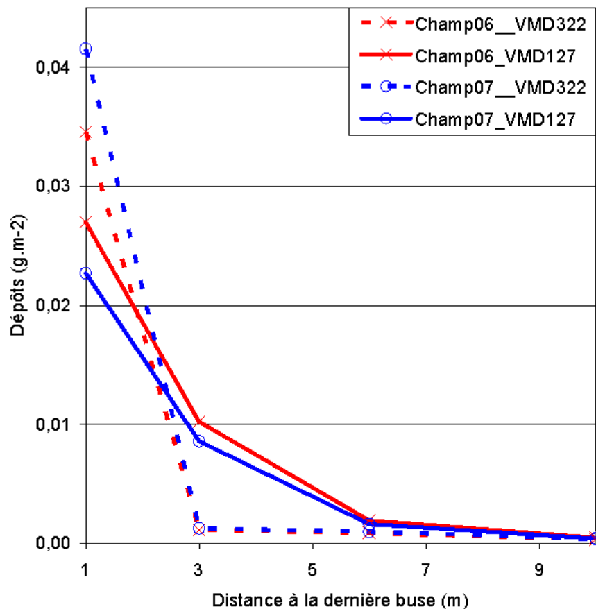
FIGURE 7.2 – Dépôts mesurés au champ pour deux VMD ( 127 et 322 \mu\text{m} ) sous différentes conditions météorologiques et rampe parallèle au vent : campagnes 2006 et 2007.
