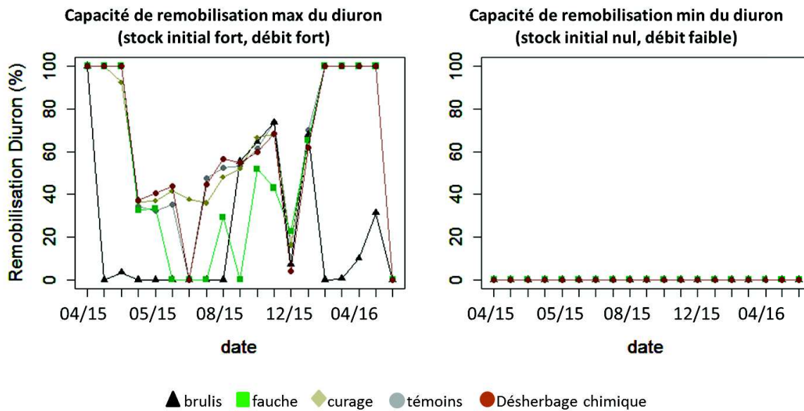
Figure 6.5 : Evolution annuelle de la capacité de remobilisation du diuron dans les biefs témoins, curés, fauchés, désherbés chimiquement et brûlés, à gauche pour le scénario combinant un stock initial de diuron maximal et une crue de période de retour d'un an et à droite pour le scénario combinant un stock initial de diuron nul et une crue de période de retour d'un mois.
