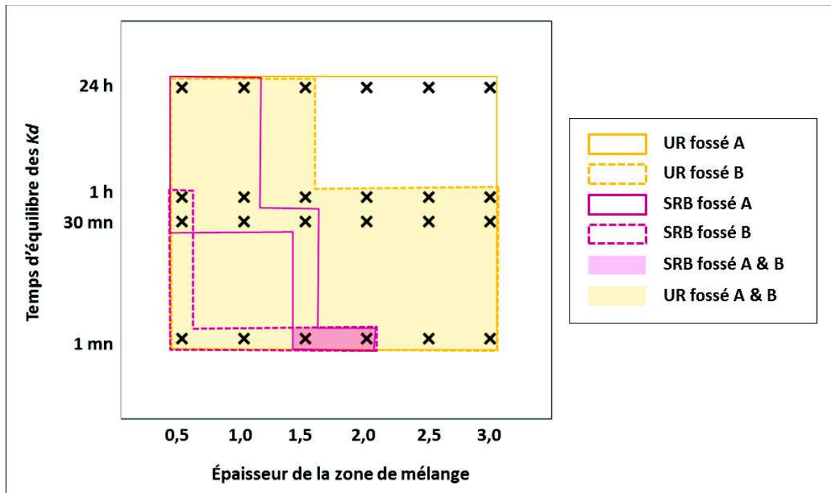
Figure 5.8 : Modèle FIP-OpenFluid - hypothèses de temps d'équilibre et d'épaisseur de zone de mélange permettant d'estimer des taux de rétention d'UR (en jaune) et SRB (en magenta) compris entre les bornes min et max des taux de rétention mesurés. Les hypothèses permettant d'estimer ces taux de rétention d'UR et SRB, respectivement, pour les deux fossés correspondent aux aires colorées en jaune pour l'UR et en magenta pour la SRB.
