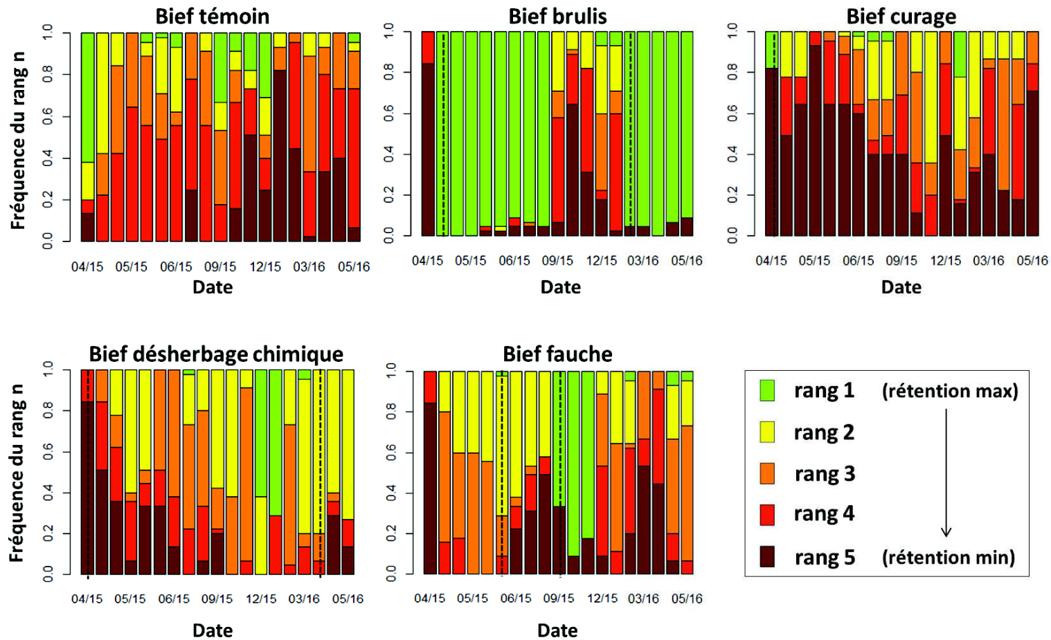
Figure 6.16 : Classement de la capacité de rétention d'herbicides (diuron, isoproturon et glyphosate) entre les biefs témoins, brûlés, curés, désherbés chimiquement et fauchés à scénarios hydrologiques et de stock initiaux équivalents. Pour un type de crue et un stock initial donné, le rang 5 est attribué au bief parmi les 5 ayant le plus fort taux de remobilisation. A l'inverse, le rang 1 un est attribué au bief ayant le plus faible taux de remobilisation. Les traits en pointillé noir représentent les opérations d'entretien.
