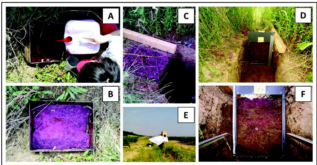
Figure 2.3 : Caractérisation de la macroporosité et des voies d'écoulement dans les sols de fond de fossé. A : infiltration de colorant dans un cadre en acier de 30 x 40 cm. B : ressuyage de la flaque. C : excavation en aval de la zone d'infiltration et mise en place d'un guide en surface. D : mise en place du cadre de prise de vue. E : tente d'ombrage pour les prises de vues. F : prise de vue du profil d'infiltration.
