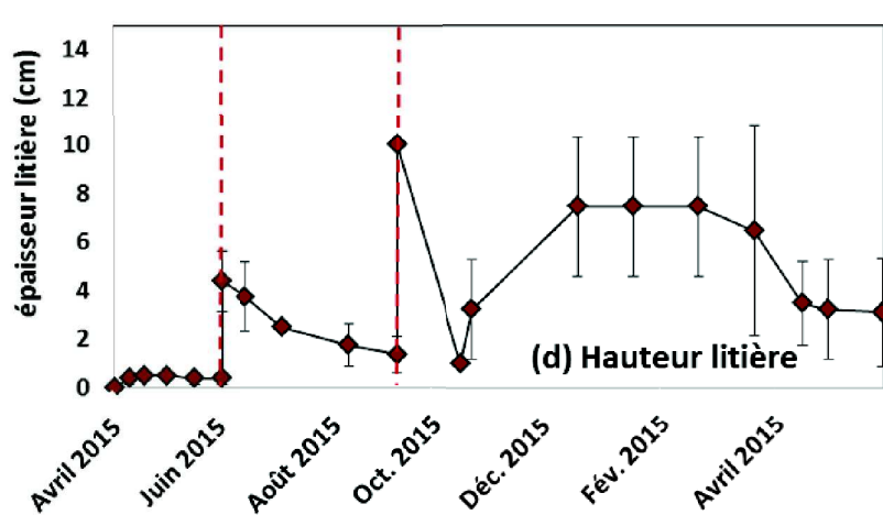
Figure 2.6 : Evolution sur les quadrats fauchés du taux de recouvrement par la végétation (a), de la classe de hauteur de la végétation (b), du taux de recouvrement par la litière (c) et de l'épaisseur de la couche de litière (d). Les barres d'erreur représentent les écarts types. Les barres en pointillées rouges représentent les opérations de fauche.
