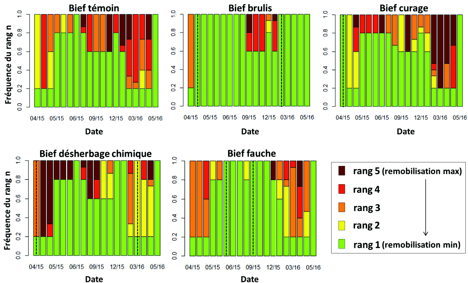
Figure 6.11 : Classement de la proportion de diuron remobilisée entre les biefs témoins, brûlés, curés, désherbés chimiquement et fauchés à scénarios hydrologiques et de stock initiaux équivalents. Pour un type de crue et un stock initial donné, le rang 5 est attribué au bief parmi les 5 ayant le plus fort taux de remobilisation. A l'inverse, le rang 1 un est attribué au bief ayant le plus faible taux de remobilisation. Les traits en pointillé noir représentent les opérations d'entretien.
