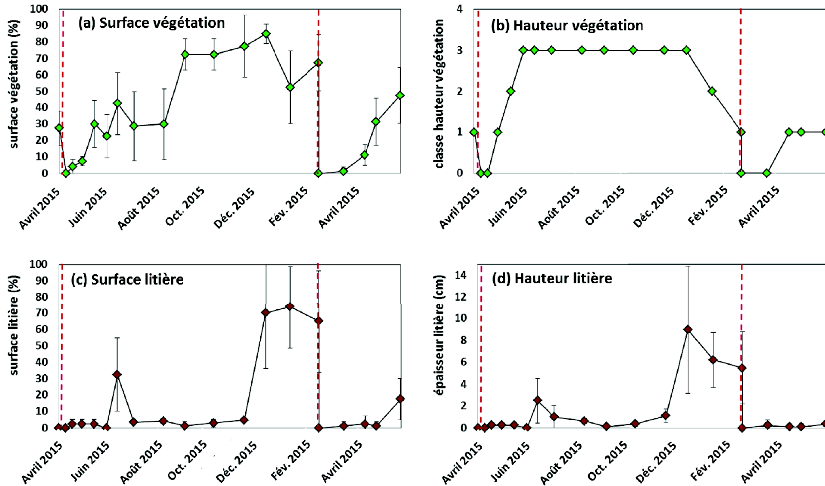
Figure 2.7 : Evolution sur les quadrats brûlés du taux de recouvrement par la végétation (a), de la classe de hauteur de la végétation (b), du taux de recouvrement par la litière (c) et de l'épaisseur de la couche de litière (d). Les barres d'erreur représentent les écarts types. Les barres en pointillées rouges représentent les opérations de brûlis.
